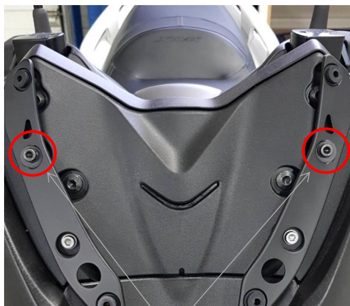
Position des vis à remplacer
